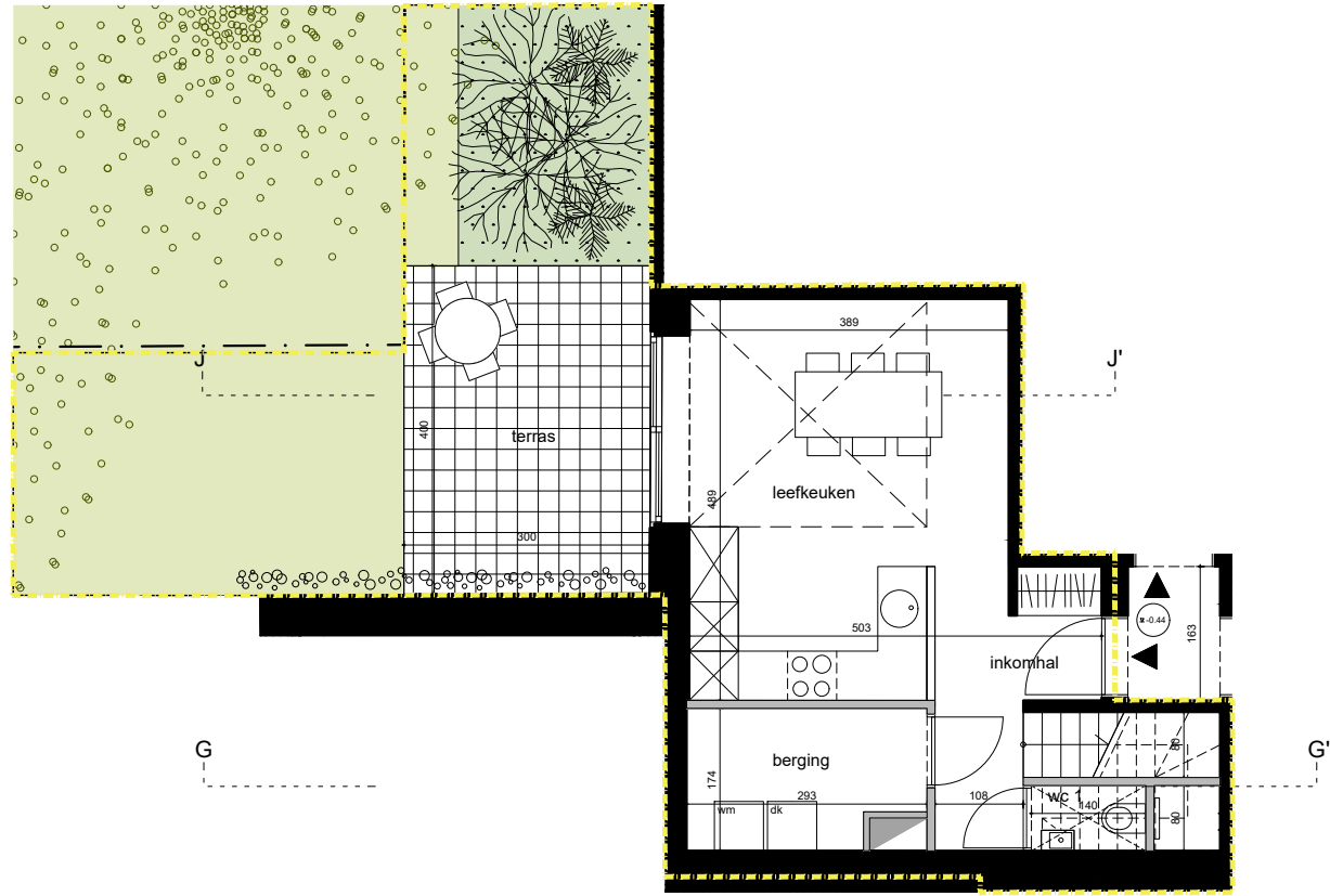
NIVEAU +0
