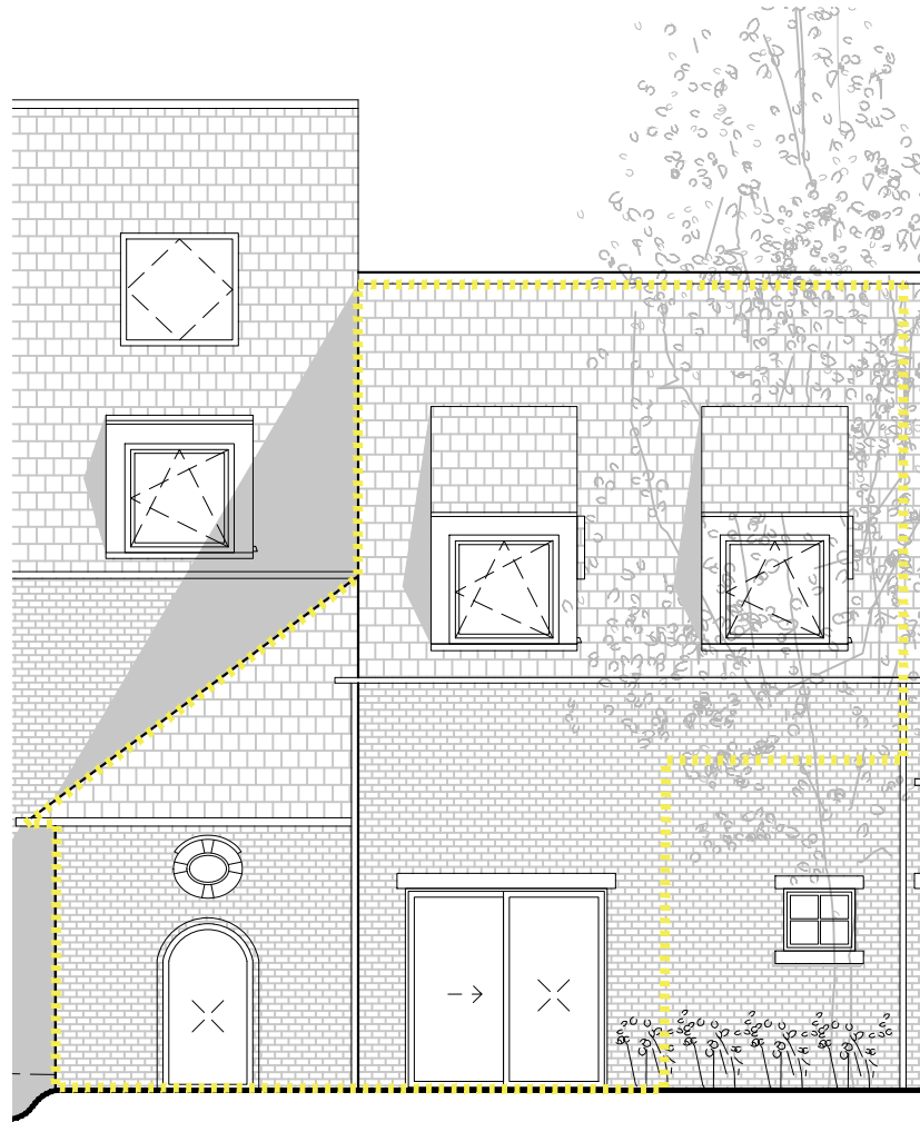
WESTGEVEL
