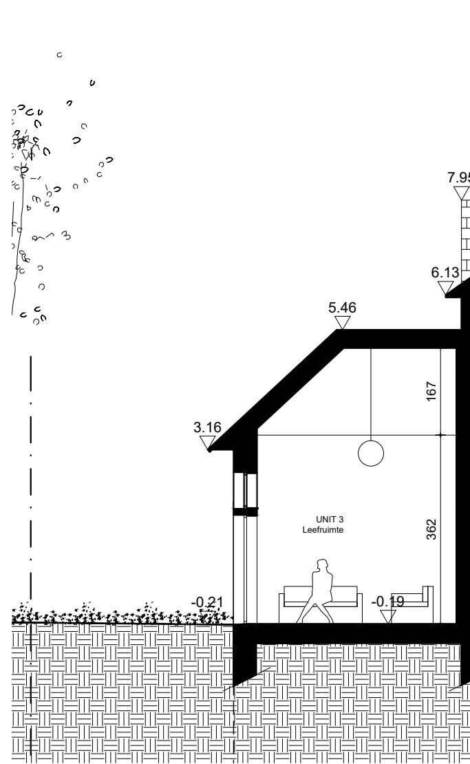
SNEDE GG'
