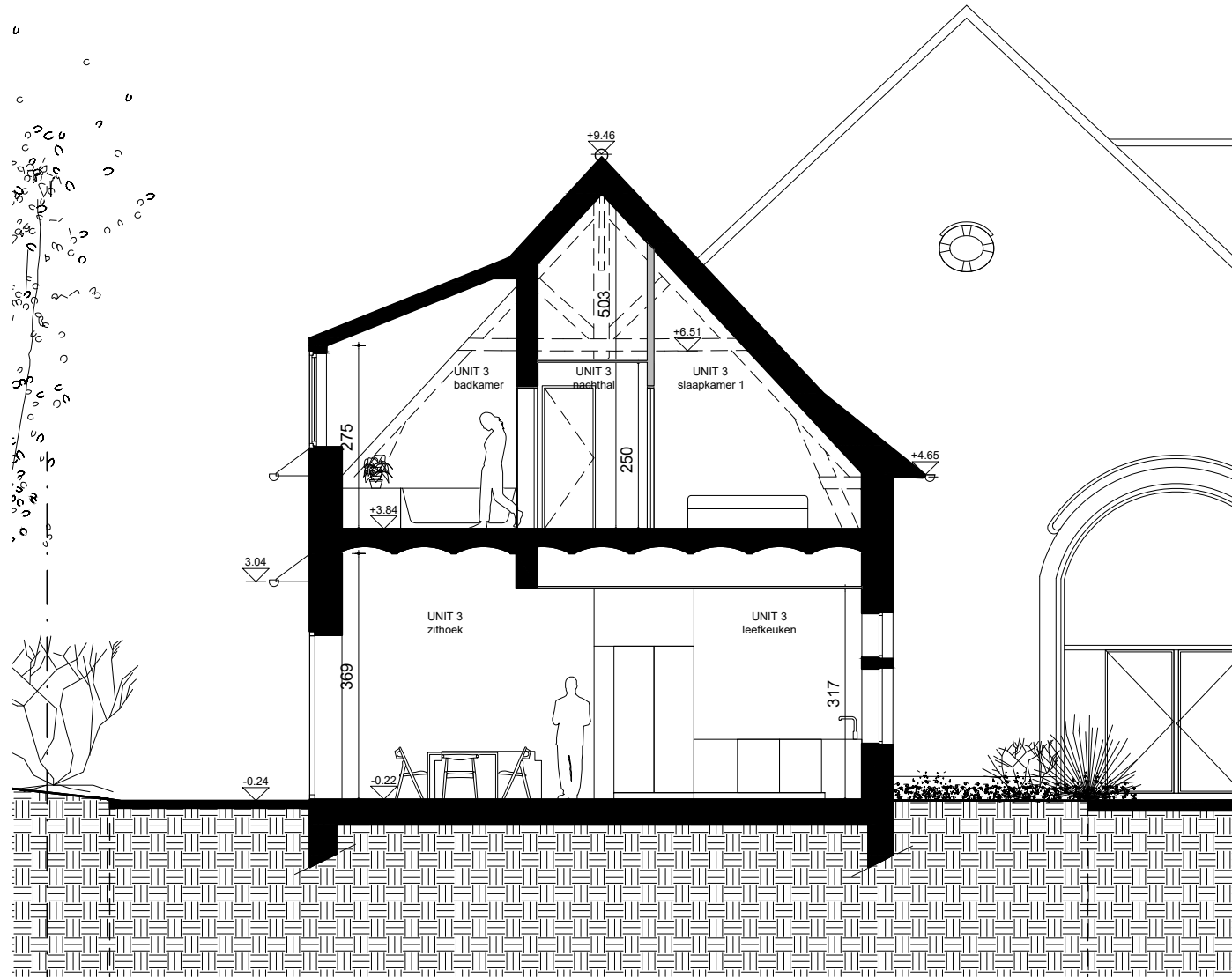
SNEDE FF'
